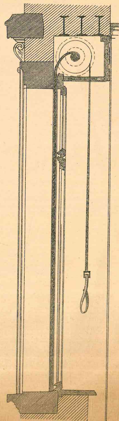
Fig. 2 - Tirante a Nastro
