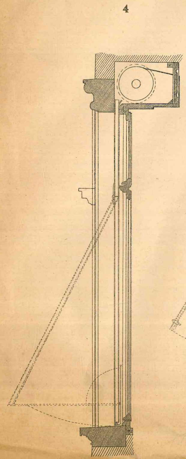
Fig. 4 - Apparecchio a sporgere N. 1 per finestre
