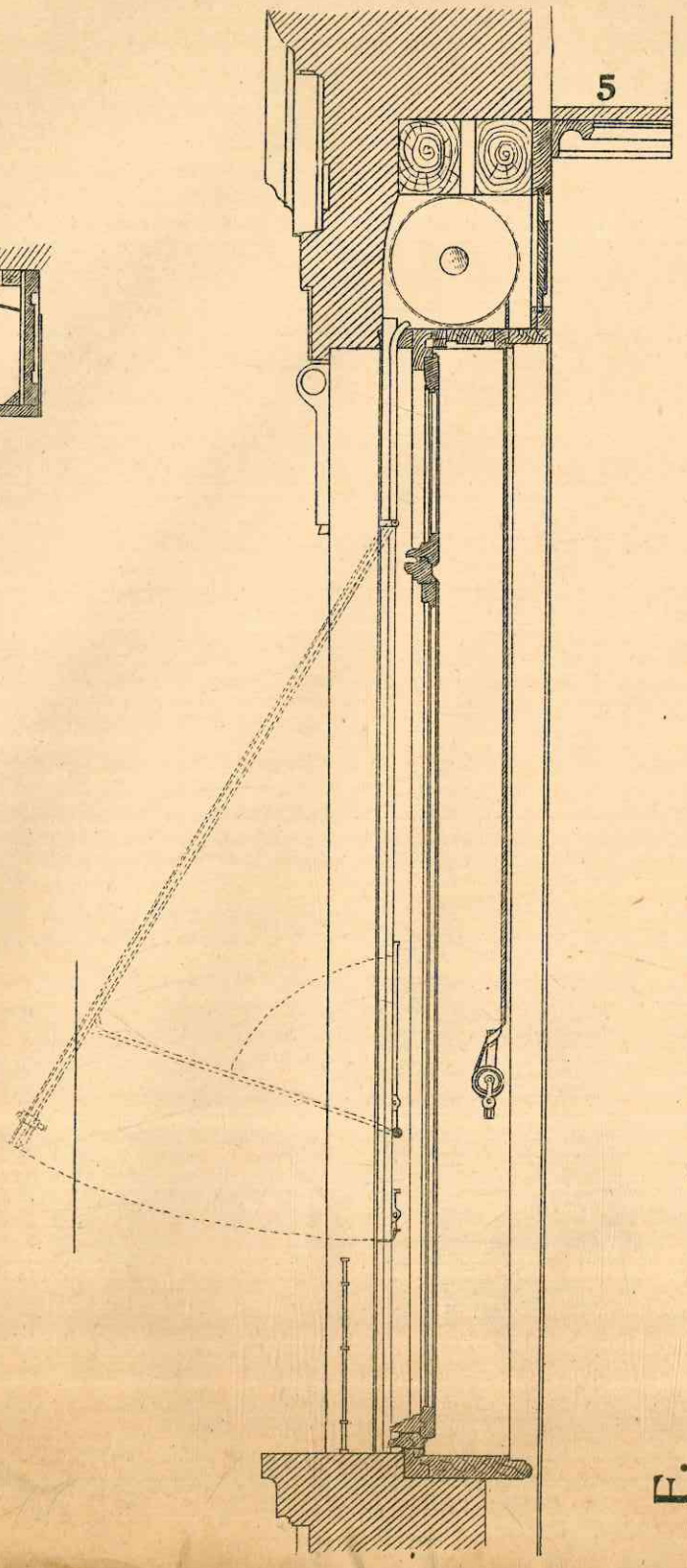
Fig. 5 - Apparecchio a sporgere N. 2 per porte e poggiatesta
