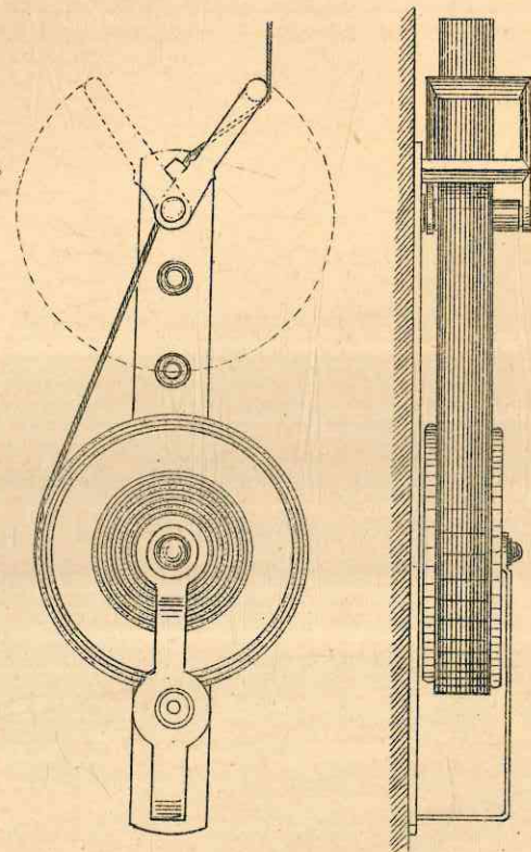
Fig. 1 - Avvolgitore automatico di cinghie d'applicarsi esternamente al muro
