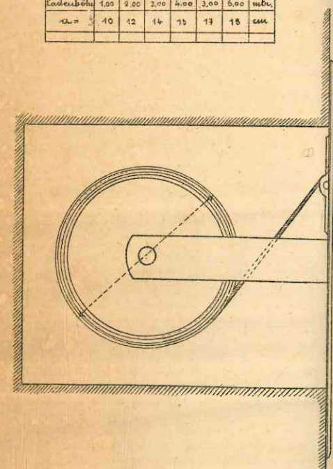
Fig. 2 - Avvolgitore automatico del da incassare nel muro
