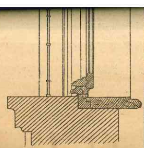
Fig. 5 - Apparecchio a sporgere N. 2 per porte e poggiuoli
