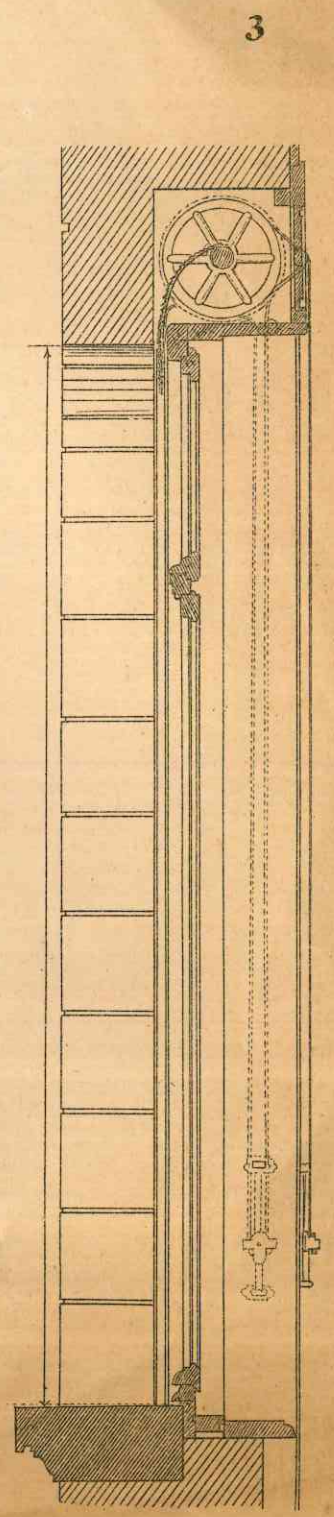
Fig. 3 Apparecchio a corda senza fine con rullo a molla Brev. 4361 con cassetta a molla laterale
