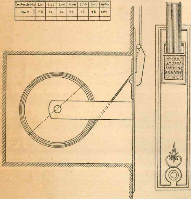
Fig. 2 - Avvolgitore automatico delle cinghie da incassare nel muro
