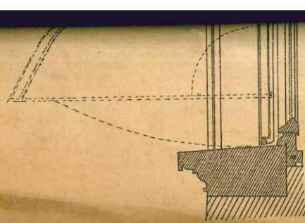
Fig. 4 - Apparecchio a sporgere N. 1 per finestre
