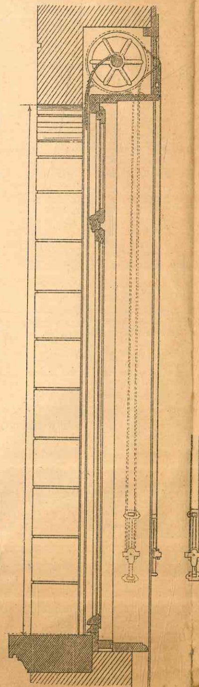
Fig. 3 - Apparecchio a corda senza fine con rullo a molla Brev. 4361 con cassetta a molla laterale
